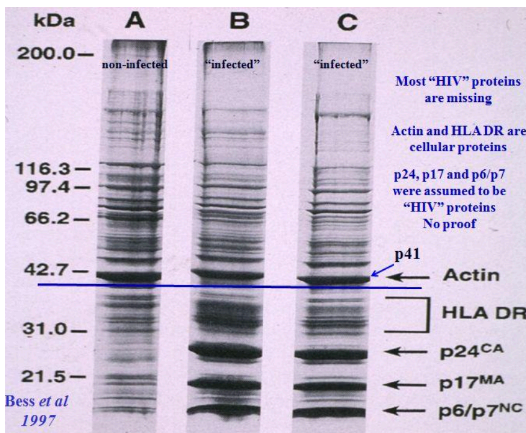
Figura 1. Bess et al., Virology , 1997 - datos de electroforesis en gel comentados por el Perth Group en 2011: A = no infectado; B, C = “infectados”.
