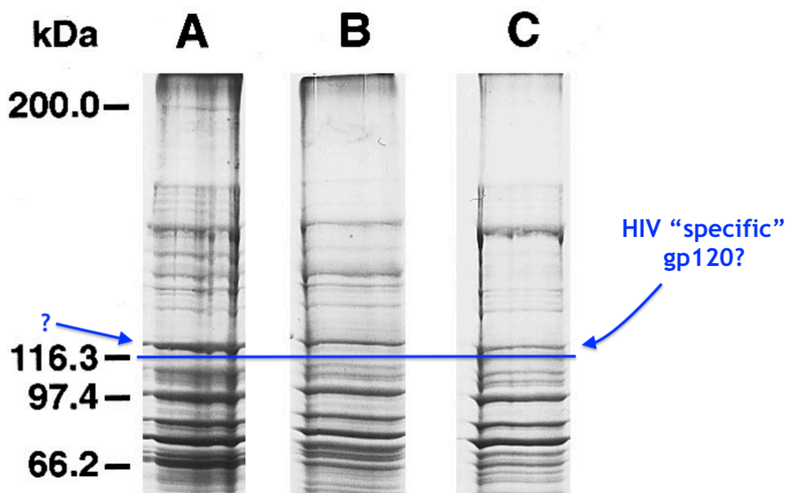
Figura 2. Bess et al., Virology 1997 - datos de electroforesis en gel enfocados por encima de la proteína marcadora de 116.3kDa : A = no infectado; B, C = “infectados”.
